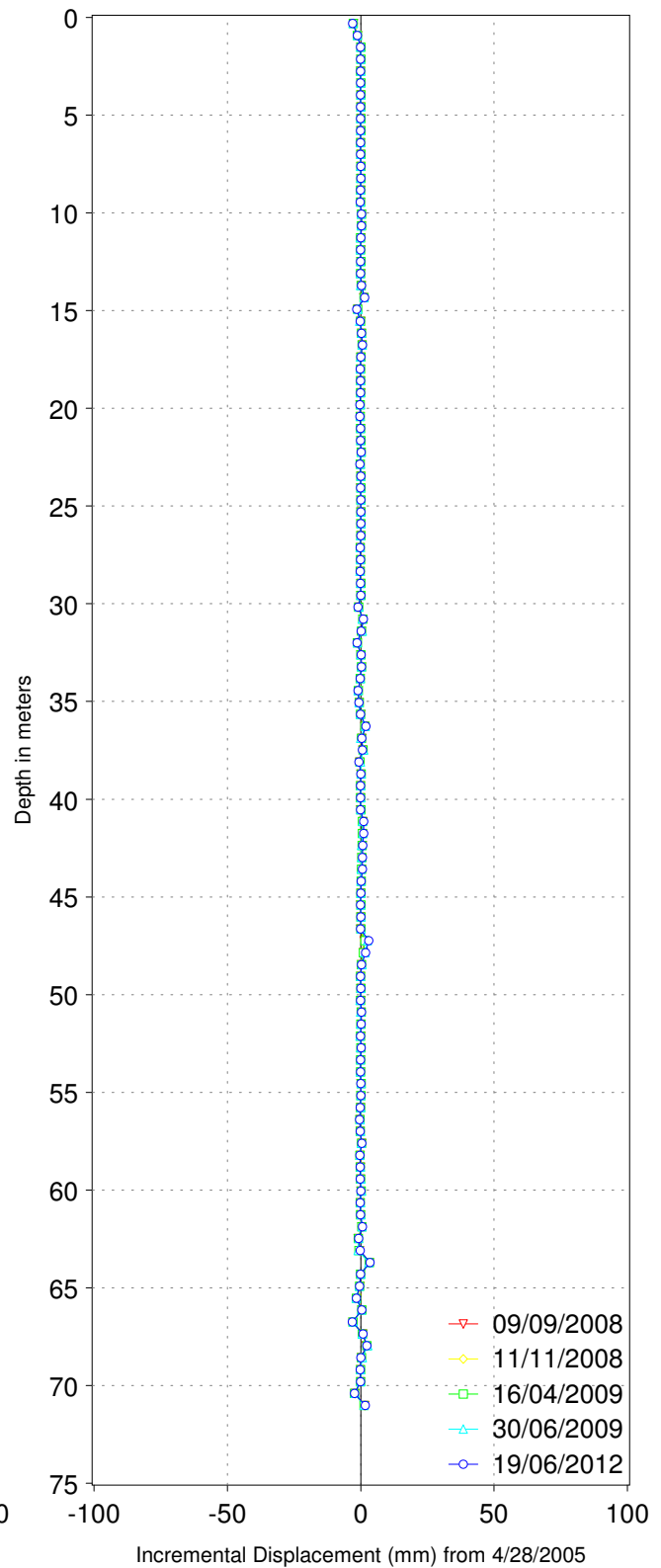
SI8, A-Axis, Incremental
